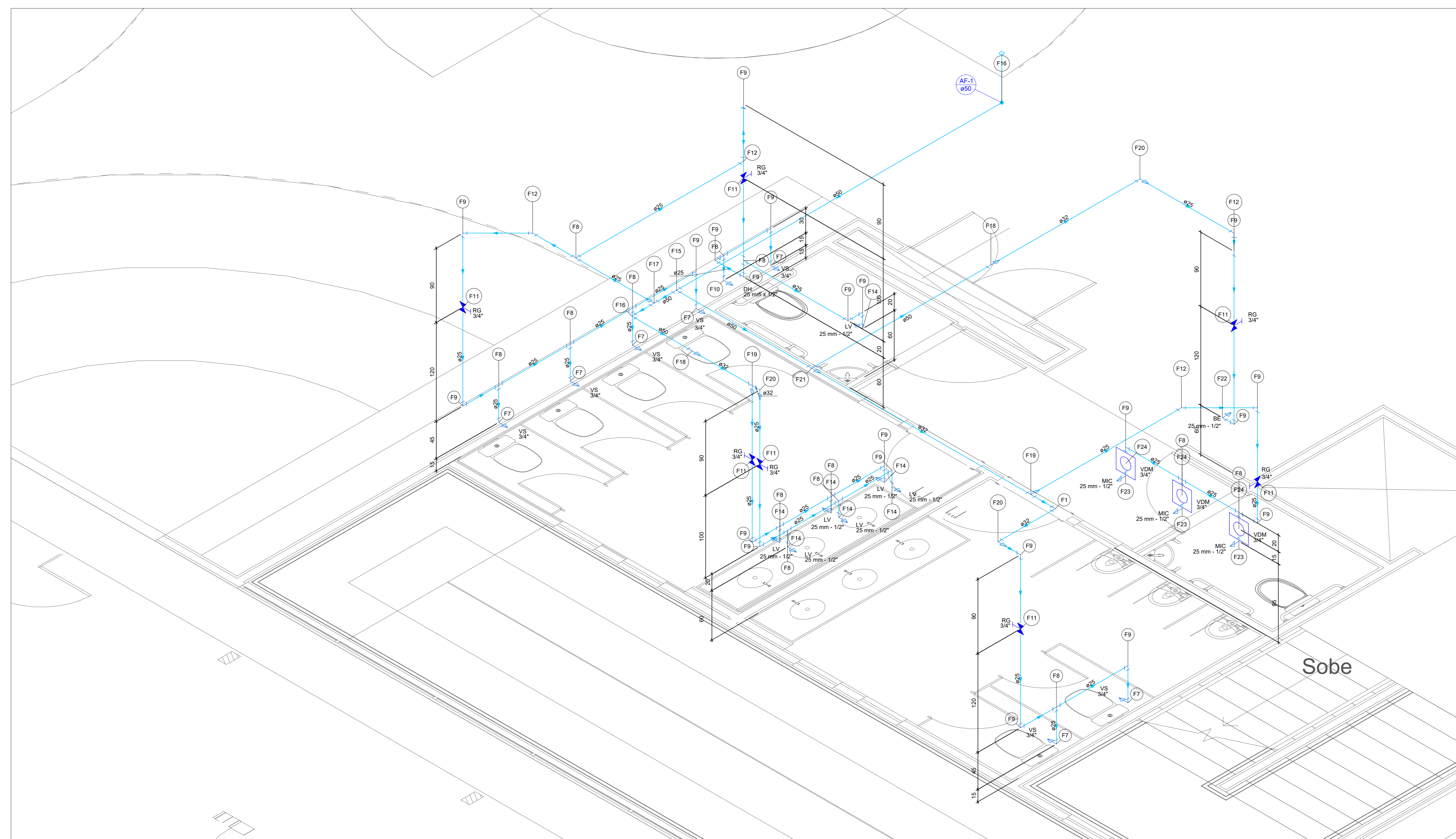
ISOMÉTRICO ESCALA: 1/25
