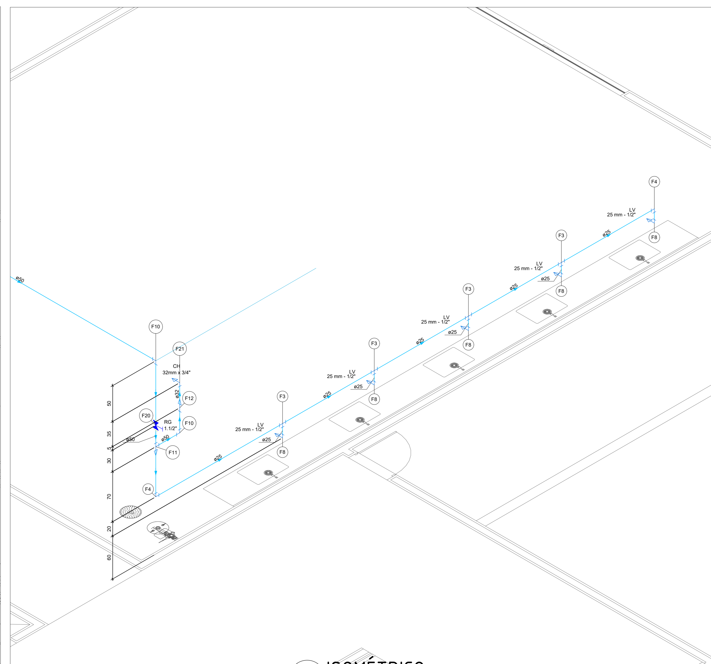
ISOMÉTRICO ESCALA: 1/25
