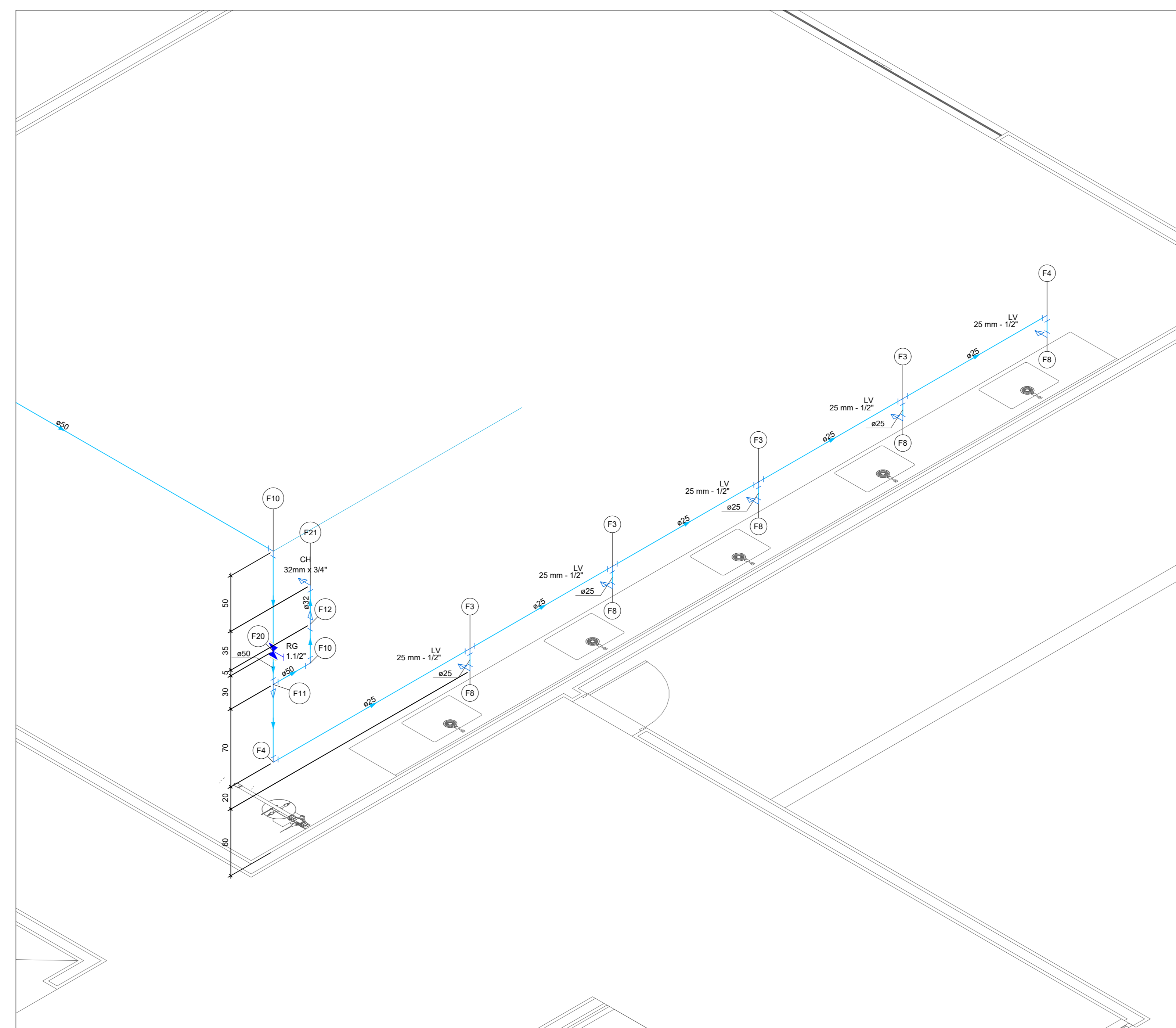
ISOMÉTRICO ESCALA: 1/25
