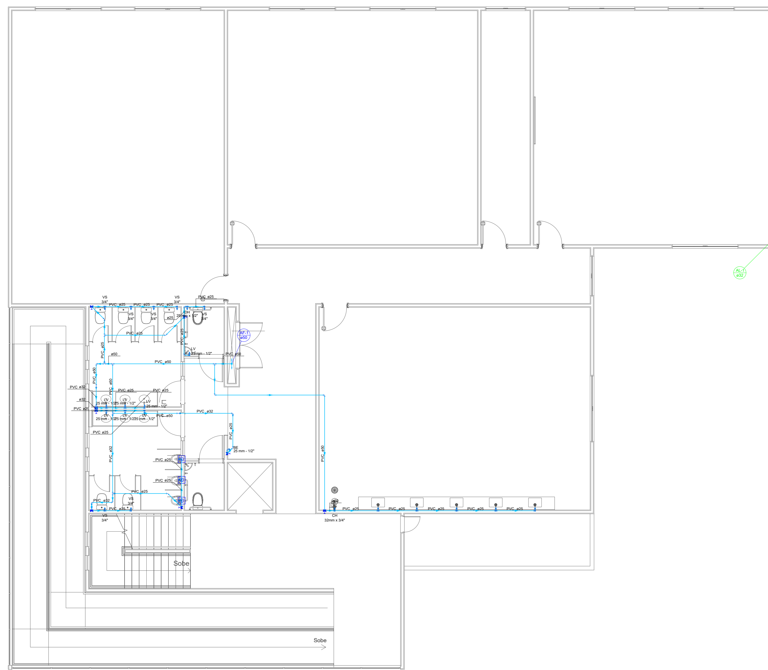
PLANTA BAIXA PAV 2 ESCALA: 1/75
